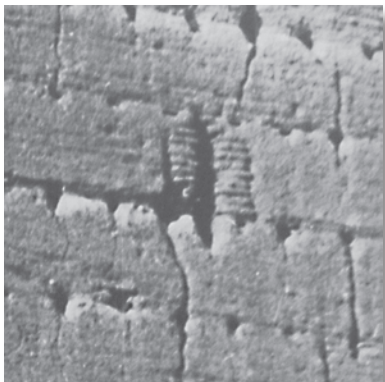
Detalle de una de los huecos o saeteras que perforan el paramento de la torre.
